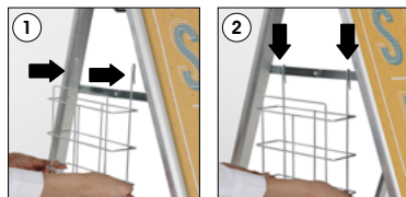
Optional Basket
